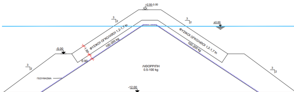
ΤΥΠΙΚΗ ΔΙΑΤΟΜΗ ΚΥΜΑΤΟΘΡΑΥΣΤΗ
